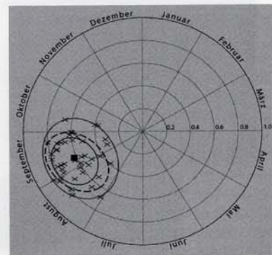
Bild 5. Illustration der «Quantilsellipsen» (90%, 75% und 50%) zur Umschreibung der zu einem Regimietyp gehörenden Stationen: Beispiel Niederwassersaisonalität für den Regimietyp 10 (pluvial inférieur). Die 90%-Ellipse ist punktiert, die 75%-Ellipse gestrichelt und die 50%-Ellipse durchgezogen eingetragen.
